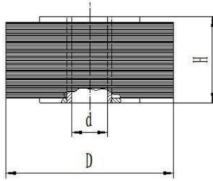
标准尺寸表 Standard Dimension
